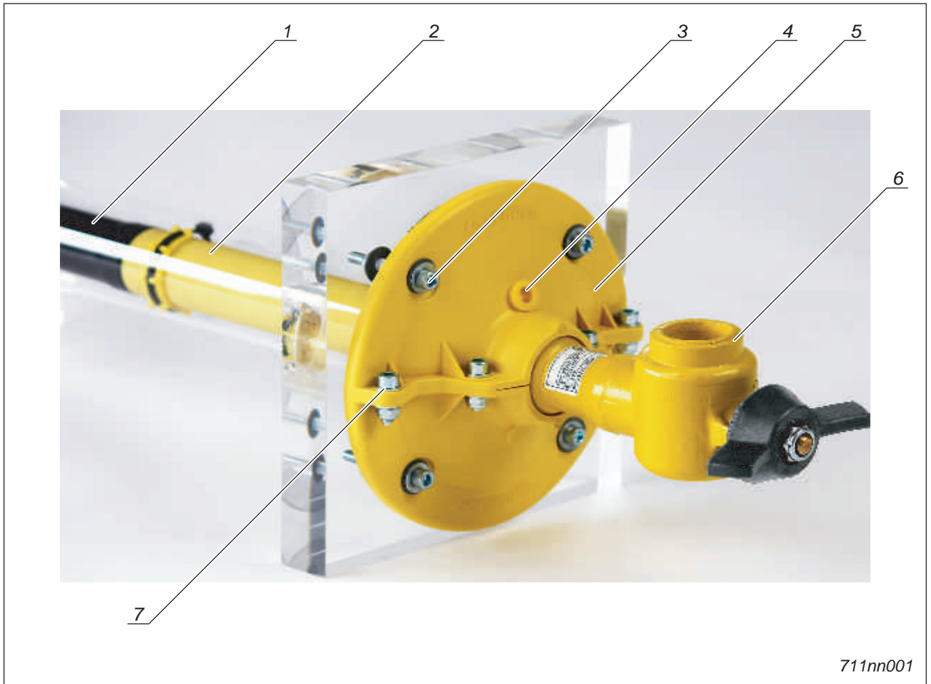
Fig. 3-1 Sanova Hauseinführung
