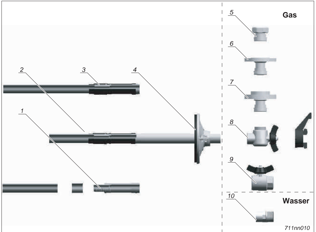
Fig. 3-2 Ausführungen Sanova Hauseinführung
