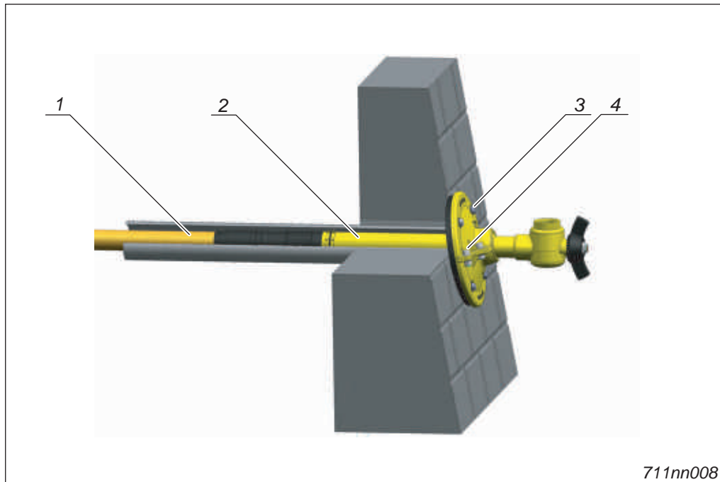
Fig. 4-2 Einbau der Sanova Hauseinführung
