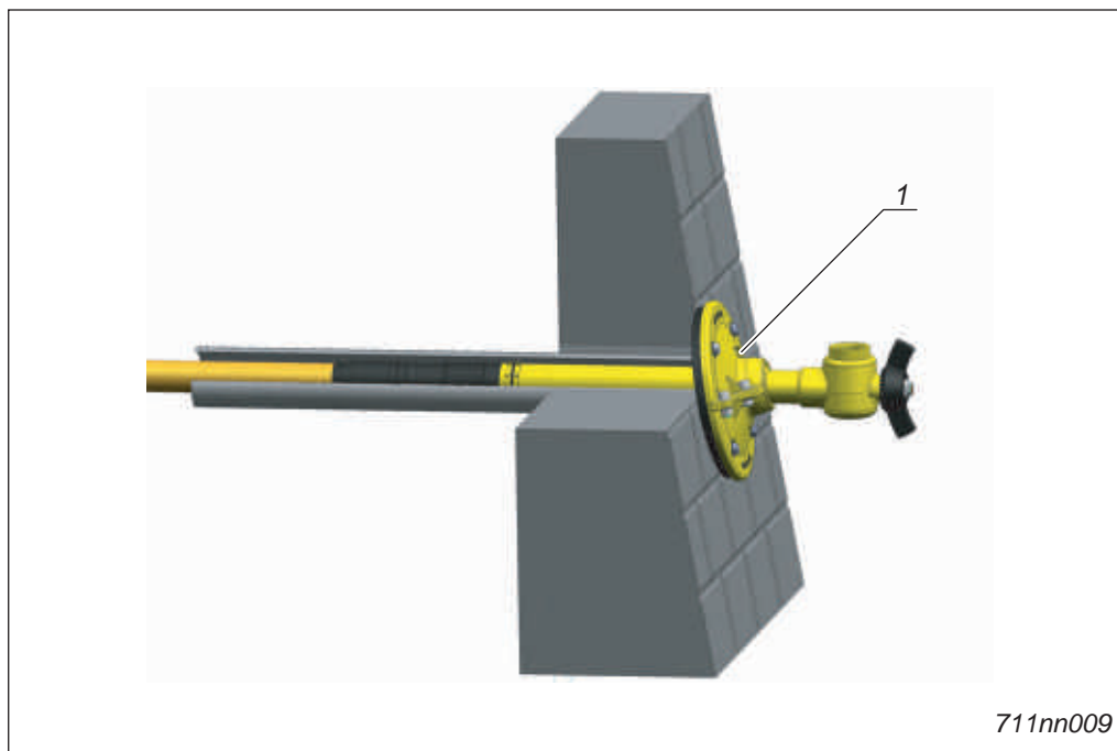
Fig. 4-3 Verdämmung Sanova Hauseinführung
