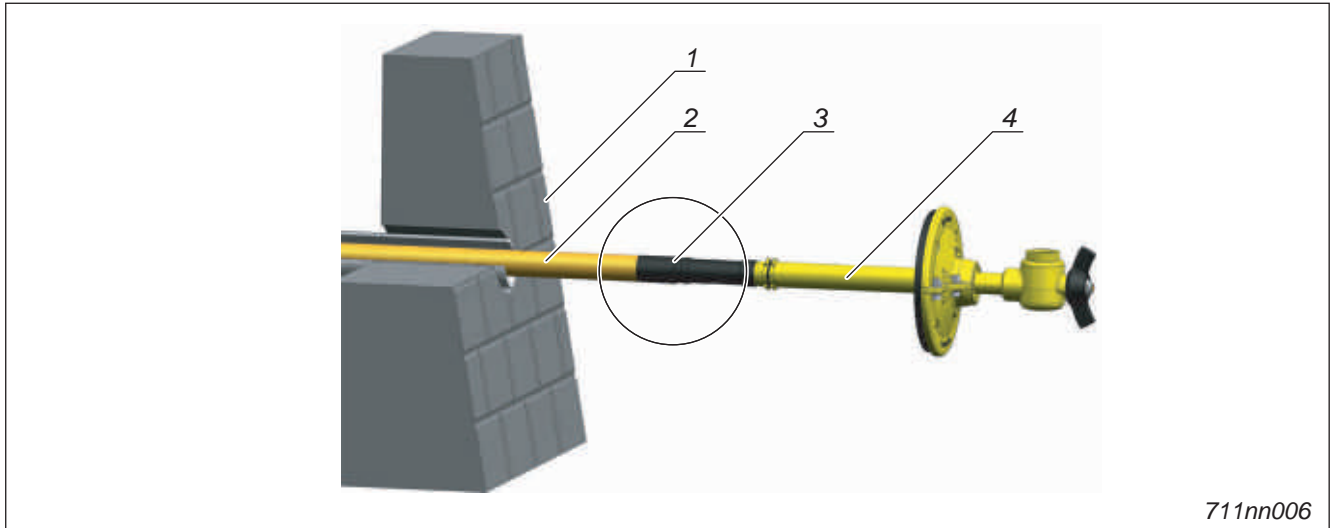
Fig. 4-1 Anschluss Sanova Hauseinführung
